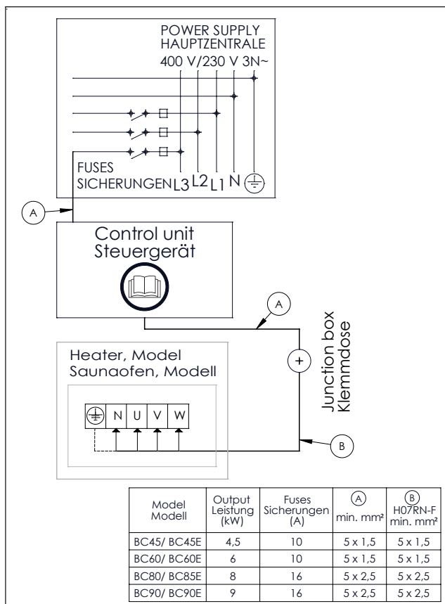
3-phase electrical connections of control unit C150 and BC-E heater 3-phasier Elektroanschlüsse des Steuergerät C150 und des Saunaofens BC-E
