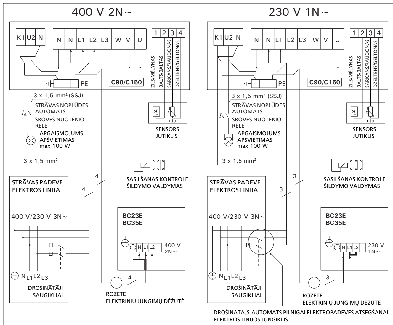
11. zīm. Elektrības pieslēgums BCE krāsnij ar C90/C150 distnces vadības pulti 11 pav. Valdymo pultis C90/C150 ir krosnelės BCE elektrinė schema
