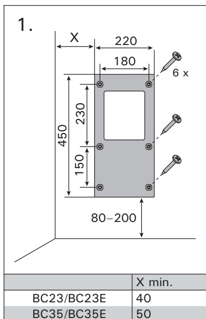
Рисунок 7. Крепление каменки к стене (все размеры приведены в миллиметрах) Joonis 7. Kerise seinalekinnitamine (kõik mõõtmed millimeetrites)
