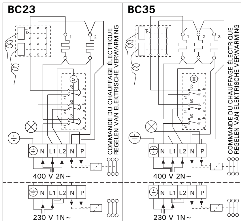
Figure 10. Raccordements électriques du poêle (BC)
