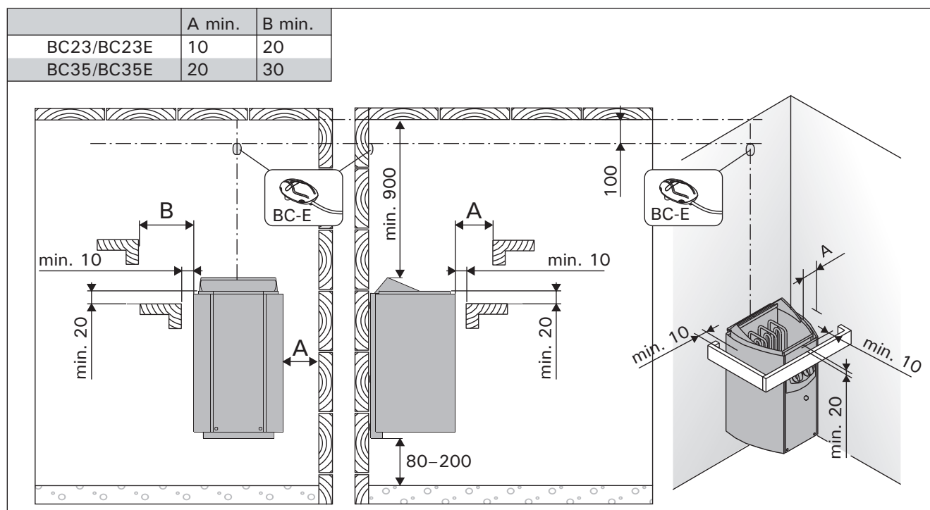
Рисунок 6. Расстояния безопасности (все размеры приведены в миллиметрах) Joonis 6. Kerise ohutuskaugused (kõik mõõtmised millimeetrites)
