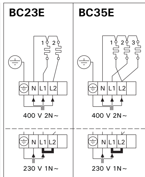
Figure 11. Raccordements électriques du poêle (BC-E)
