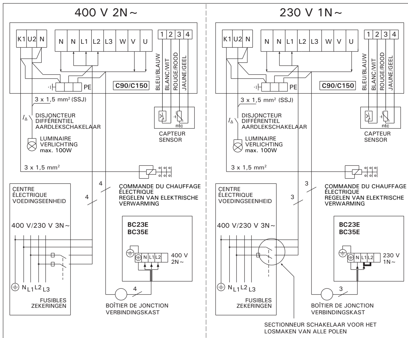
Figure 11. Centre de contrôle C90/C150 et raccords électriques du poêle BC-E
