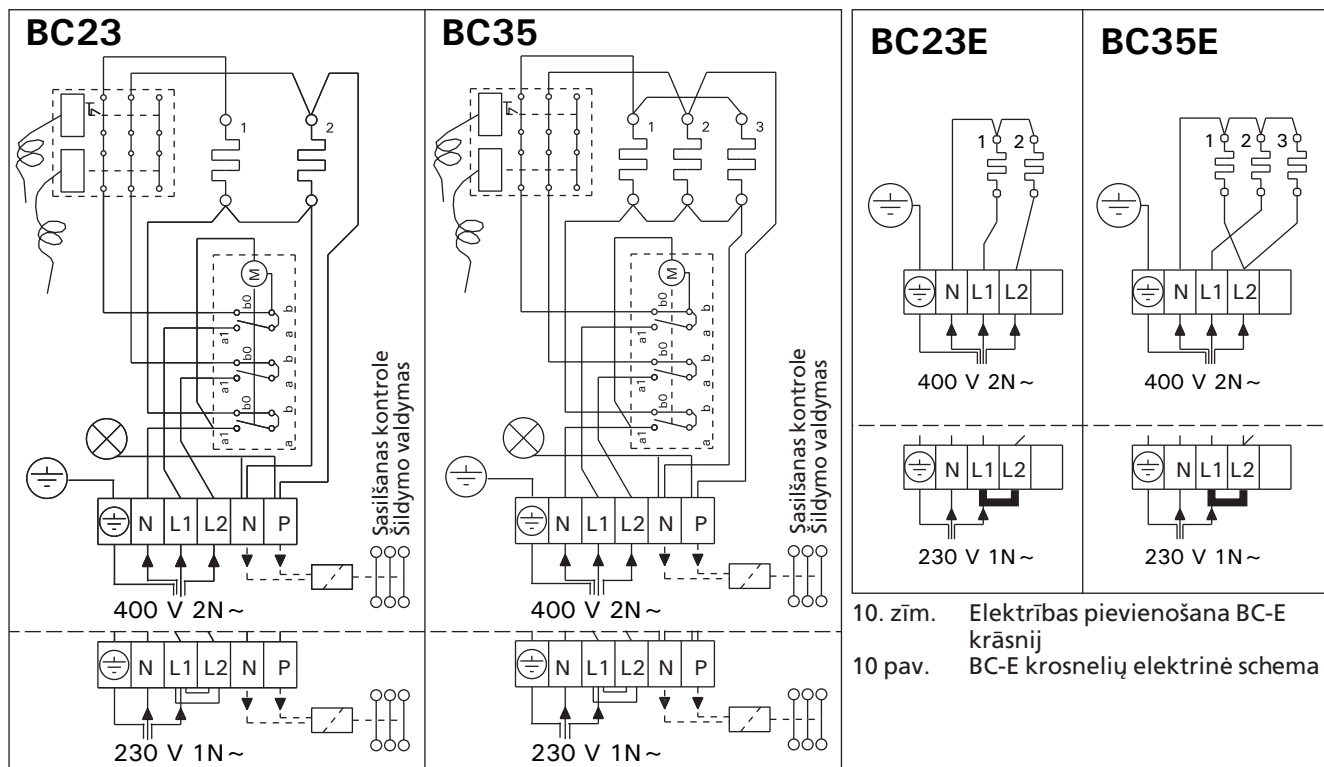
9. zīm. Elektrības pievienošana BC krāsnij 9 pav. BC krosneliņu elektrinė schema
