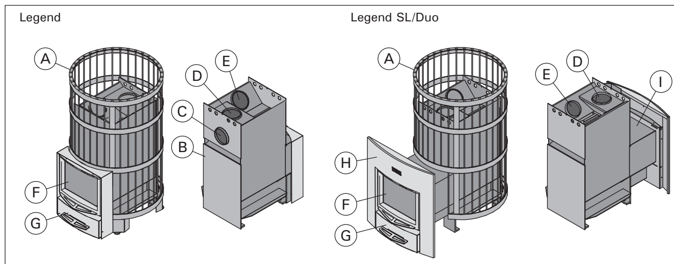
Рисунок 1. Элементы конструкции каменки. Внимание! Используйте только запасные части, рекомендованные изготовителем каменки. Несанкционированная модификация каменки запрещается. Joonis 1. Kerise osad. Tähelepanu! Kasuta ainult tootja poolt heakskiidetud varuosi. Keriste loata ümberehitamine on keelatud.
