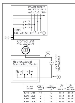
3-phase electrical connections of control unit C150 and BC-E heater 3-phaseser Elektroanschlüsse des Steuergeräts C150 und des Saunaofens BC-E
