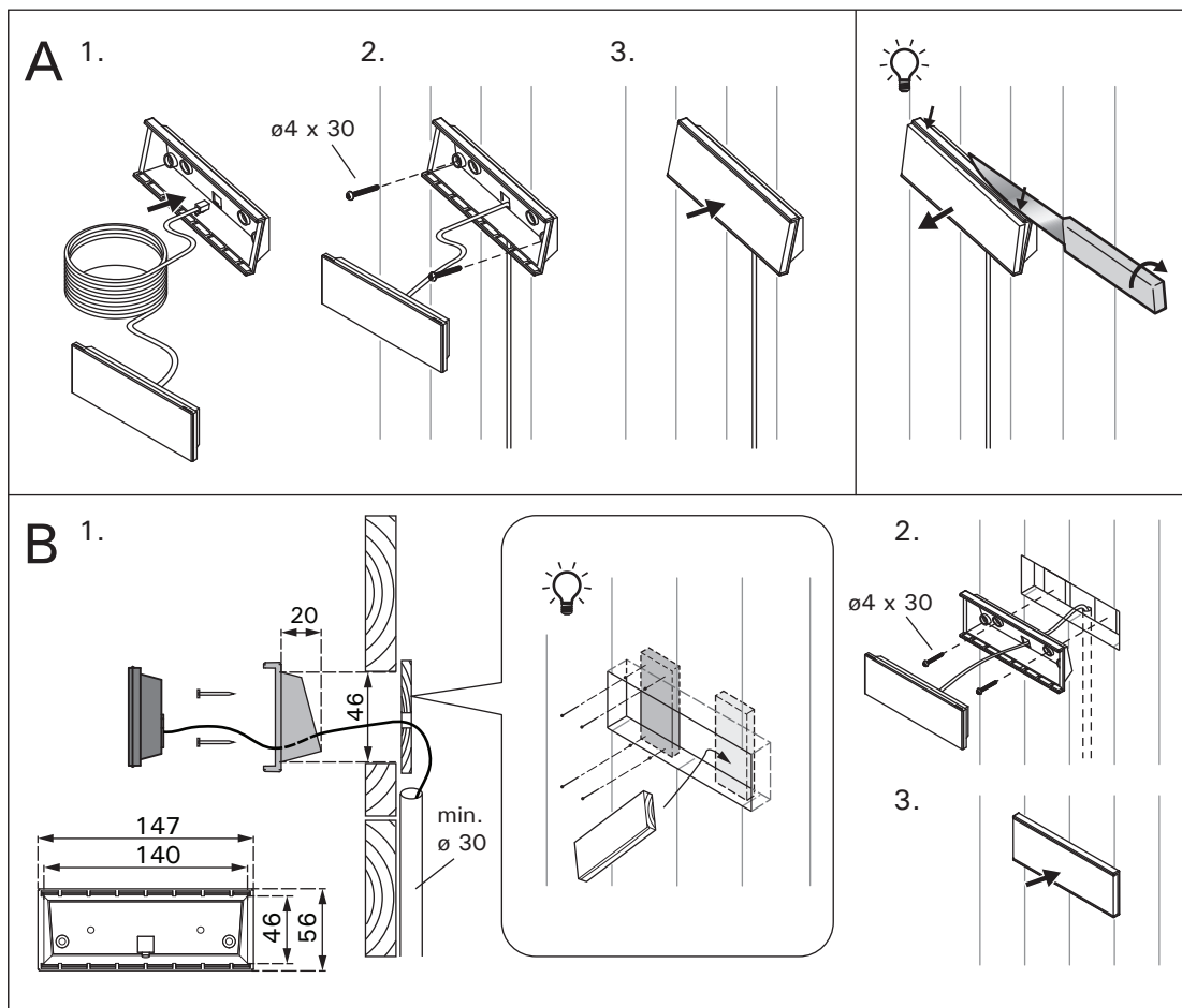
Figura 8. Cómo fijar el panel de control
