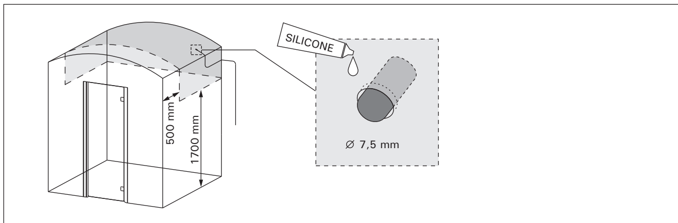
Kuva 5. Lämpöanturin sijoittaminen
