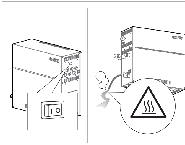
Kuva 2. Sakkakupin tyhjennys Bild 2. Tömning av slamkopp
