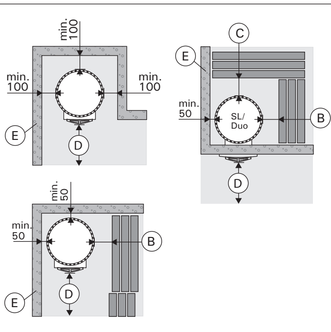
Рисунок 9. Безопасные расстояния (все размеры приведены в миллиметрах)
