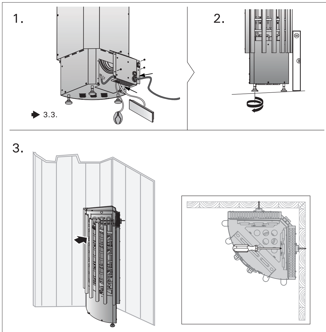
Figure 8. Installing the heater Abbildung 8. Installation des Saunaofens
