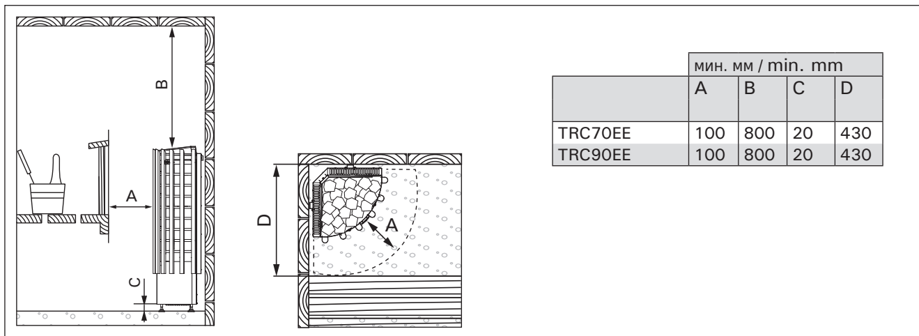
Рисунок 4. Расположение и безопасные расстояния (все размеры приведены в миллиметрах)
