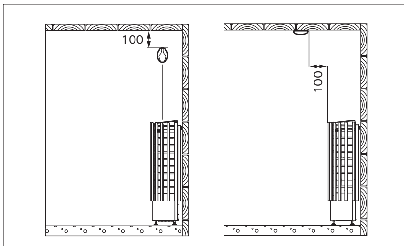
Kuva 6. Anturin asentaminen (mitat millimetreinä)
