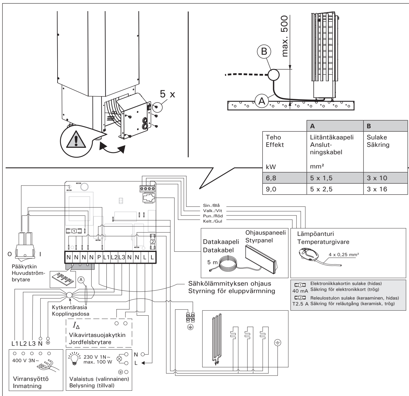
Kuva 5. Sähkökytkennät Bild 5. Elnstallationer
