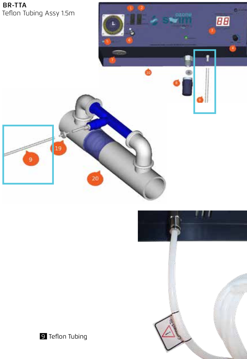
Teflon Tubing
