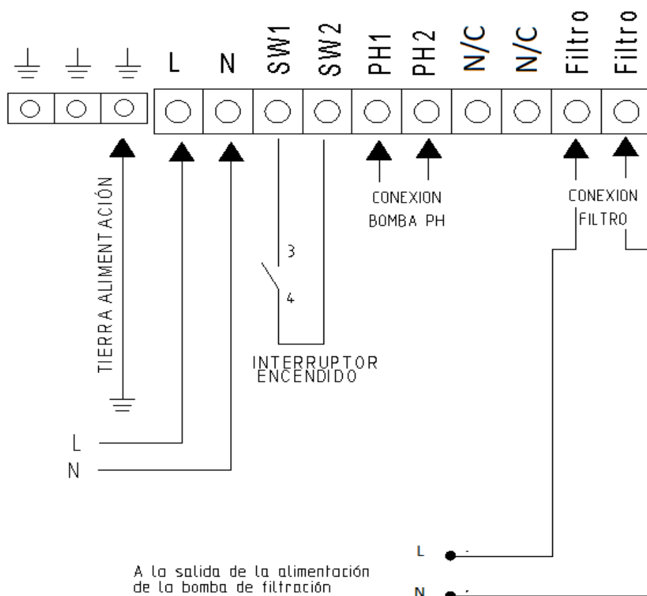
CONEXIÓN CONTROL MARCHA – PARO
