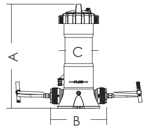
MODEL: CL-01A & CL-02A (Off-line)
